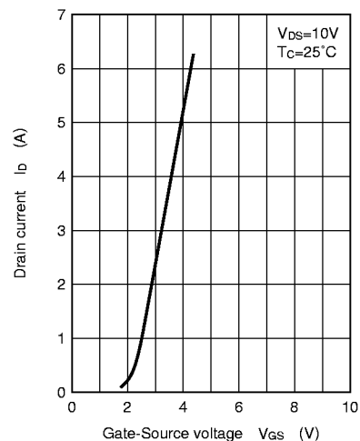
I_D - V_{GS}
