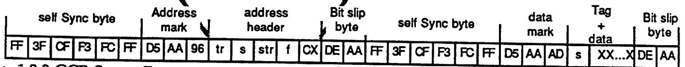
Fig. 1.3.3 GCR Sector Format
