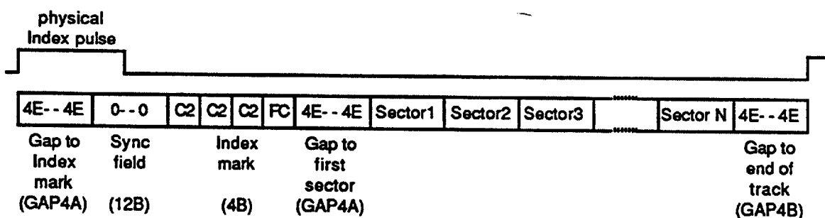
Fig. 1.3.2.1 MFM Track Format
