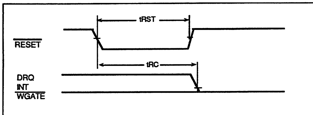
Fig. 9 Negative Reset
