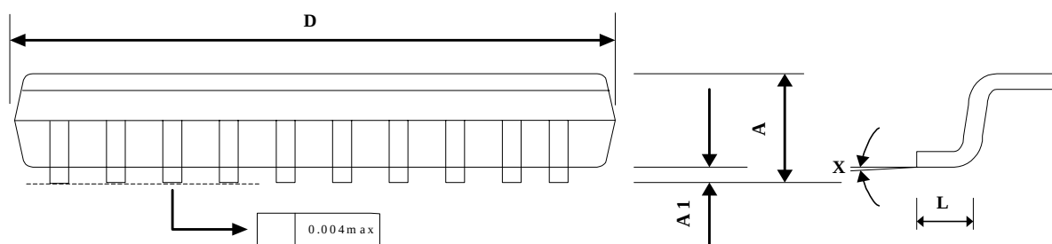
20-LEAD
