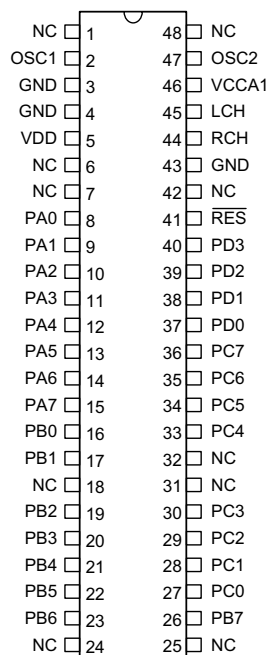
HT36A0 - 48 DIP-A
