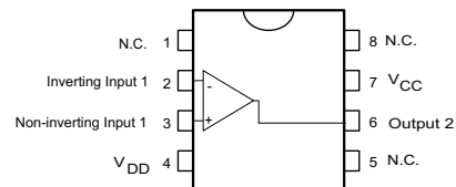
TS942ID-TS942IDT-TS942IPT
