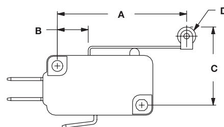
FIG. 2 Lever Roller
