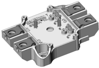
SEMiX® 1s
