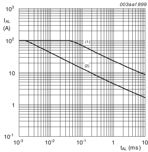
(1) T_{j (avr)} = 25^{\circ}C ; (2) T_{j (avr)} = 100^{\circ}C
