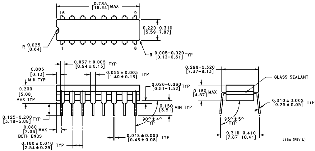
16-Lead Ceramic Dual-In-Line Package (D) NS Package Number J16A
