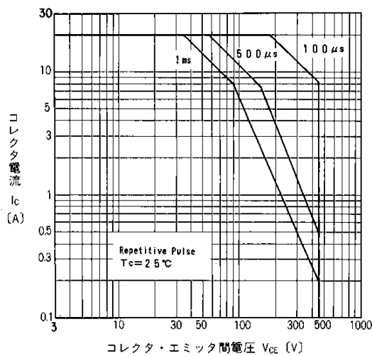
安全動作領域特性(線返し) Safe Operating Area
