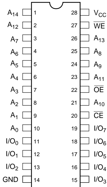
28-Pin SOJ
