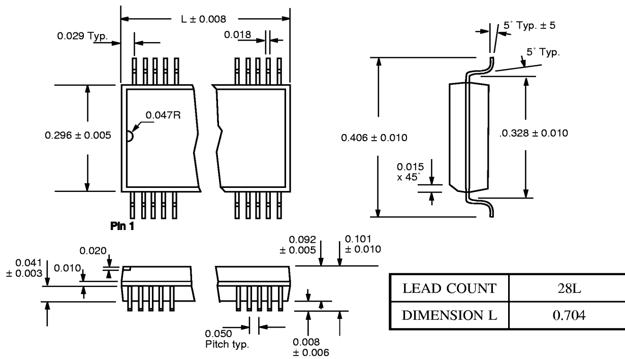
SOIC Package
