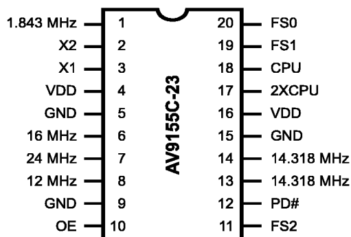
20-Pin DIP or SOIC
