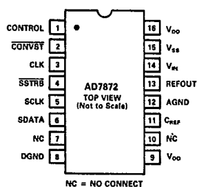
DIP, SOIC
