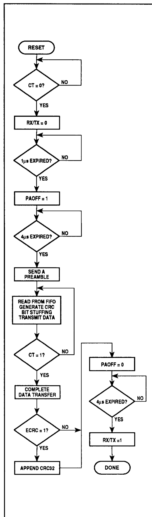
Fig. 13 Data transmit
