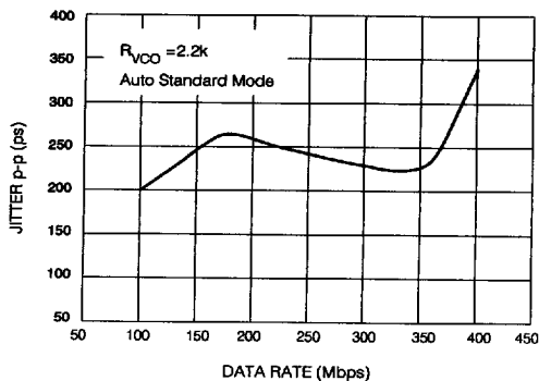
Fig. 5 Output Jitter
