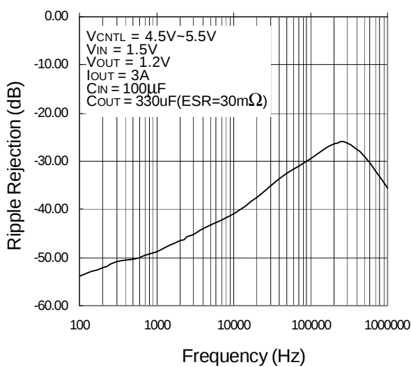
VCNTL PSRR
