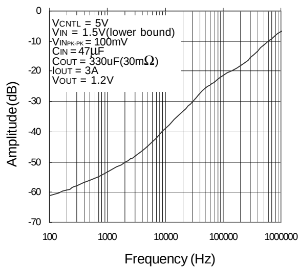
VIN PSRR
