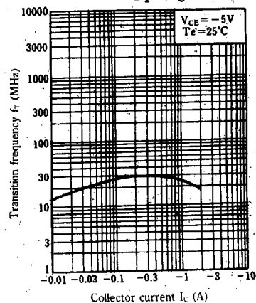
f_T - I_C
