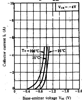
I_C - V_{BE}
