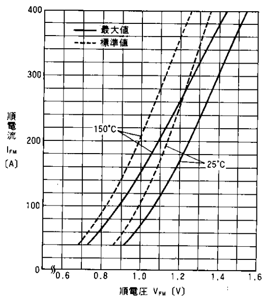
順特性
