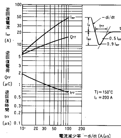
逆回復特性
