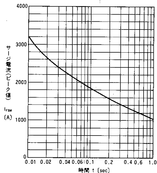
サージ電流
