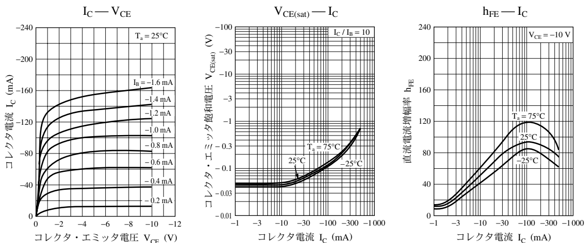
UNR112X特性図
