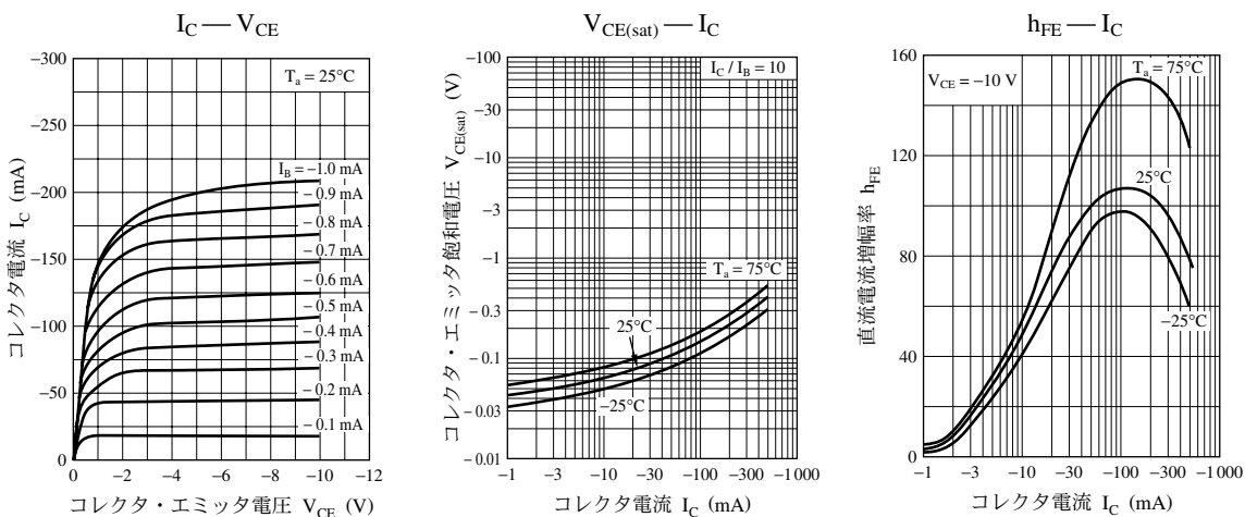
UNR1122 特性図
