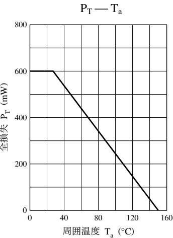
共通特性図
