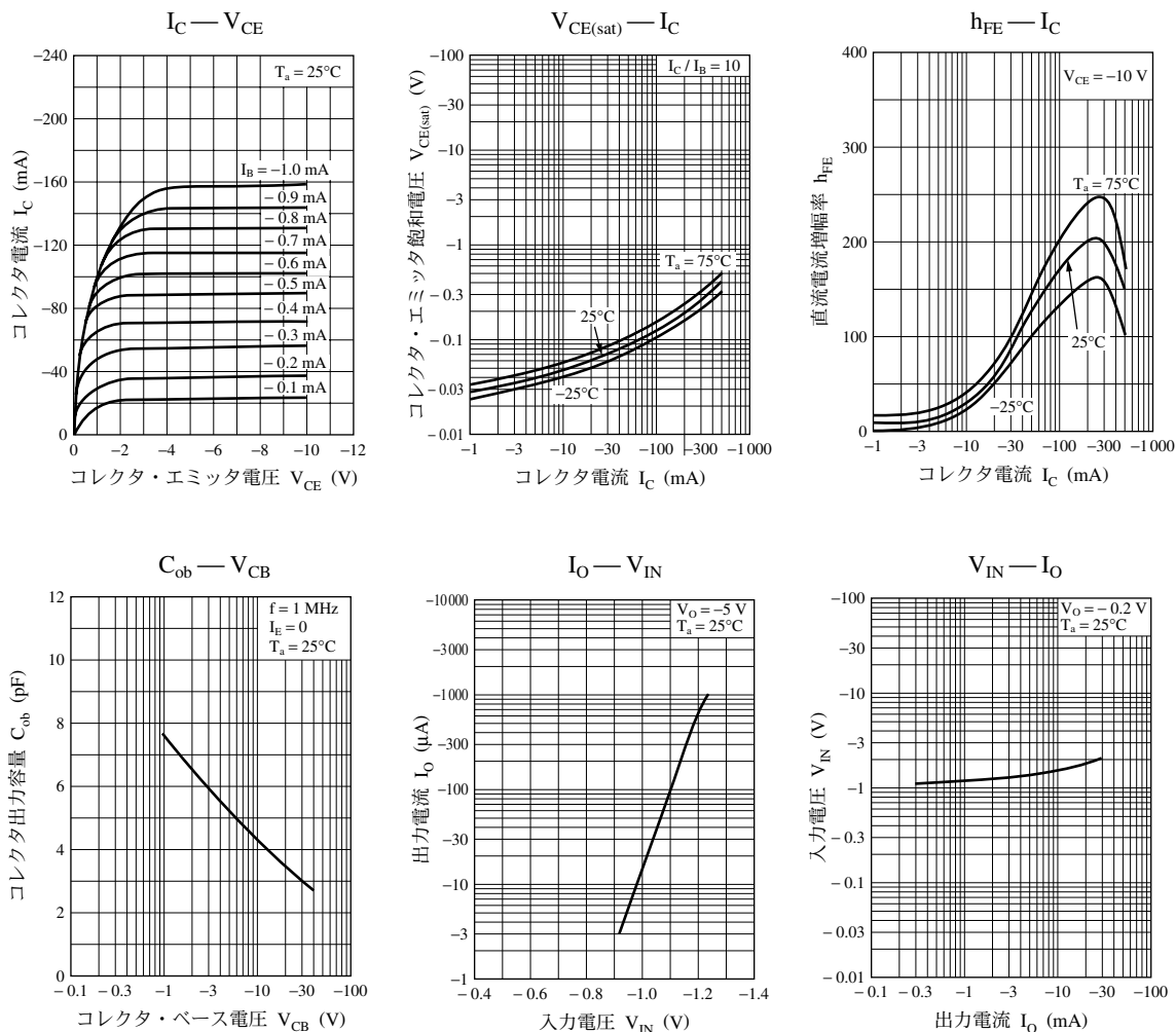
UNR1121 特性図
