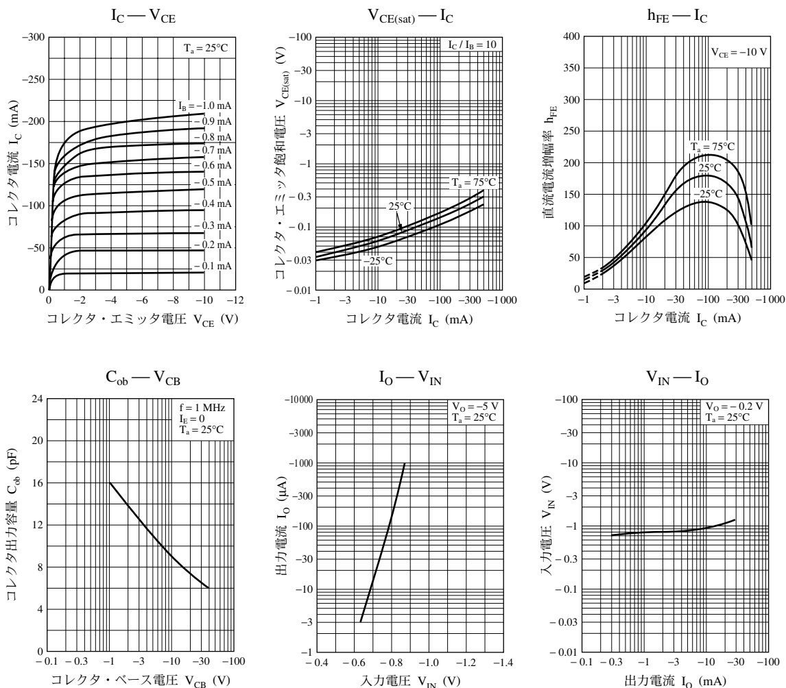
UNR1124特性図
