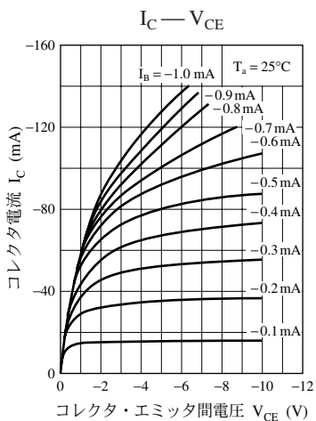
UNR1112 特性図
