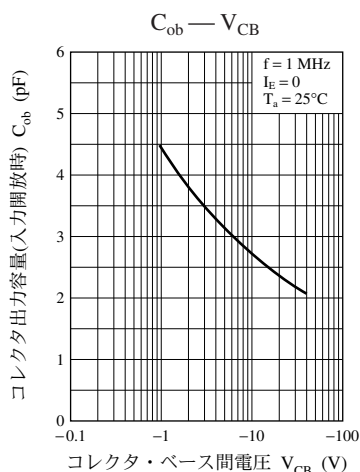
UNR1115 特性図
