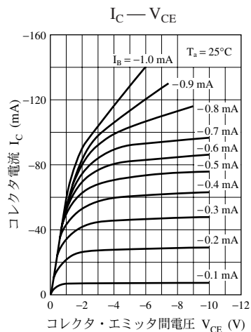
UNR1111 特性図
