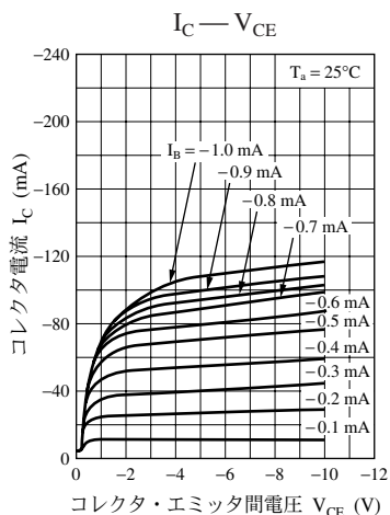
UNR1118 特性図
