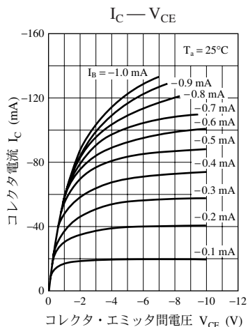
UNR1114 特性図
