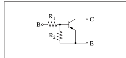
内部接続図
