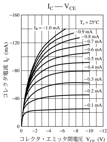
UNR1115 特性図
