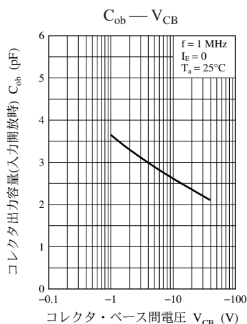
UNR1118 特性図
