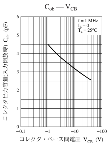
UNR1112 特性図
