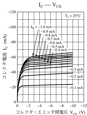
UNR1117 特性図
