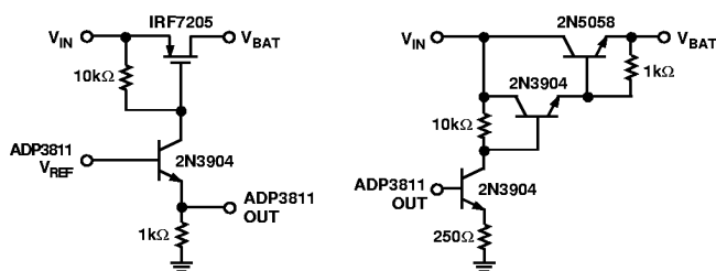
a. P-Channel MOSFET
