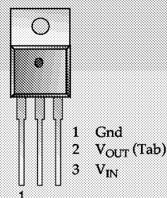
3L TO-220 Tab ( V_{OUT} )
