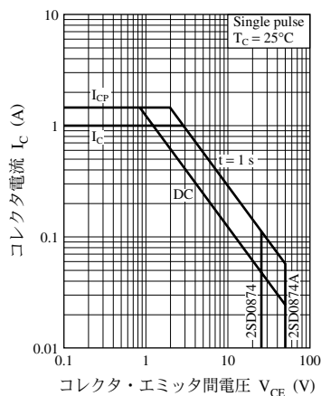
安全動作領域
