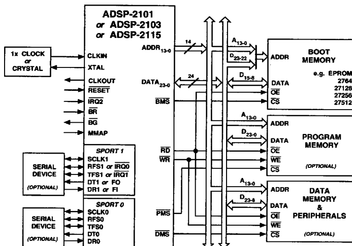
Figure 3. ADSP-2101/ADSP-2103/ADSP-2115 System
