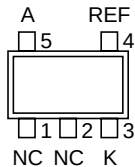
MPAK-5 (HA17L431LP/ALP)
