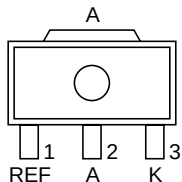
UPAK (HA17L431UP)
