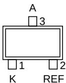
MPAK (HA17L432ALTP)
