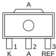
UPAK (HA17L432UP)
