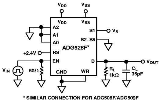
Test Circuit 9. Enable Delay, t_{ON} (EN) , t_{OFF} (EN)
