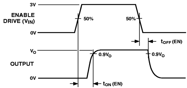
Test Circuit 9. Enable Delay, t_{ON} (EN) , t_{OFF} (EN)
