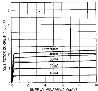
Fig. 4 出力特性
