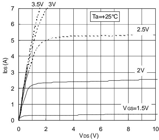
V DS -I DS CHARACTERISTICS
