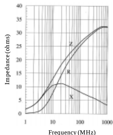
BMB-1J-0025P-S2
