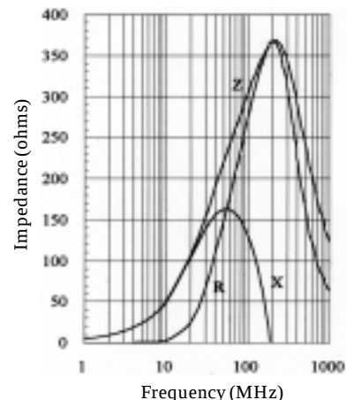
BMB-1J-0060-N2
