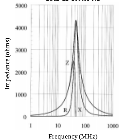
BMB-2B-2000A-N2
