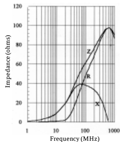
BMB-2A-0300L-N2
