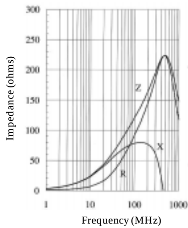
BMB-2B-0120M4-N2
