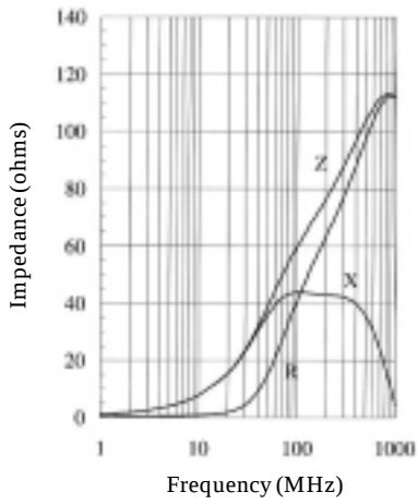
BMB-2B-0060M4-N2
