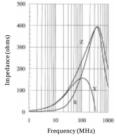
BMB-2B-0240M4-N2
