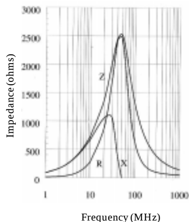
BMB-2B-2000A-N1
