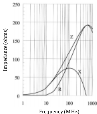
BMB-2J-0120P-N2
