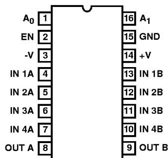
HI1-539 (CERDIP) HI3-539 (PDIP) TOP VIEW
