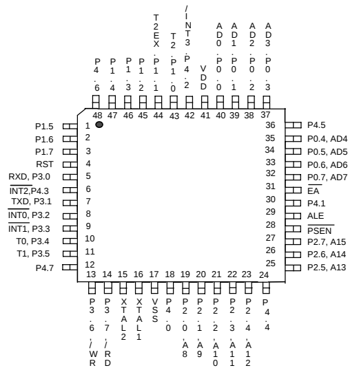
48-Pin LQFP (W78E365D)
