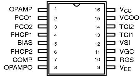
16 Pin SOIC
