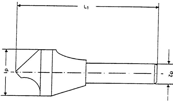
Kegel- und Entgratsenker mit Querloch 90° in Kunststoffkassette Slotted taper and deburring countersinkers 90° in polystyrene case
