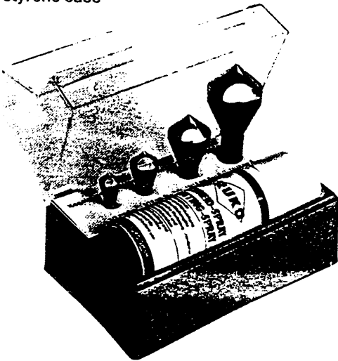
Kegel- und Entgratsenker mit Querloch 90° in Kunststoffkassette Slotted taper and deburring countersinkers 90° in polystyrene case
