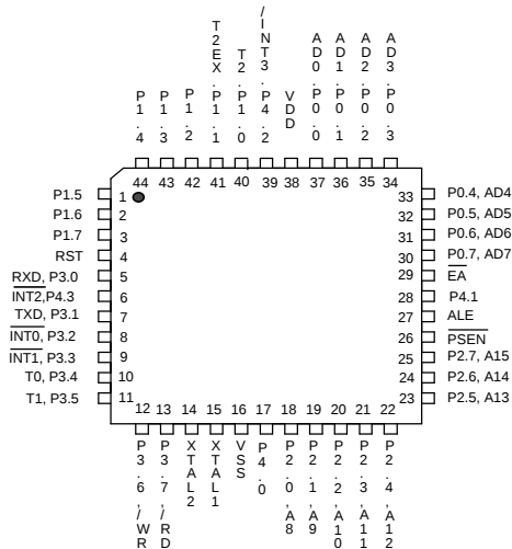
44-Pin PQFP (W78E365F)
