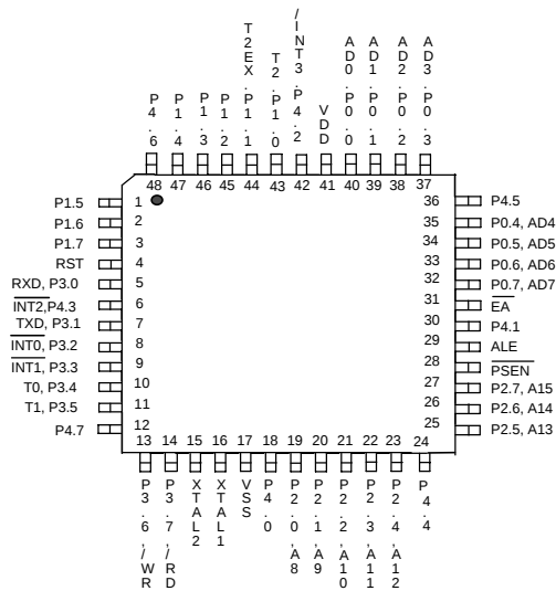
48-Pin LQFP (W78E365D)
