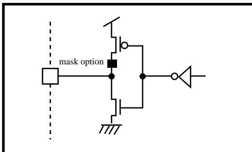
TYPE I/O
