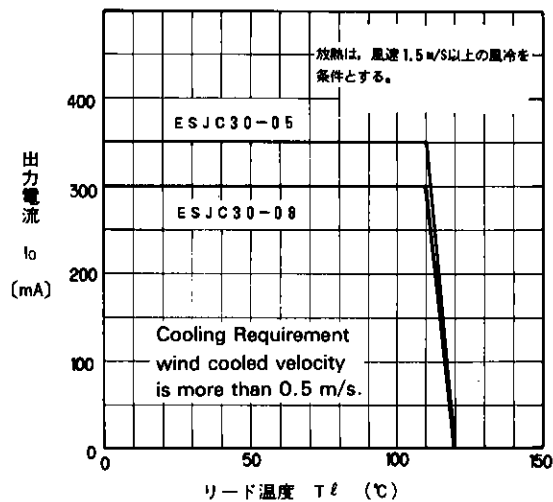
電流低減特性曲線 Current Delaying Curve
