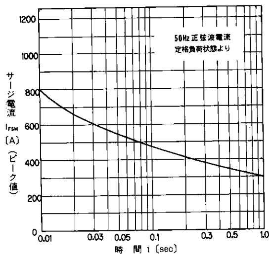
サージ電流 Surge Current
