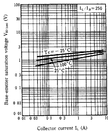
V_{BE(sat)} - I_C
