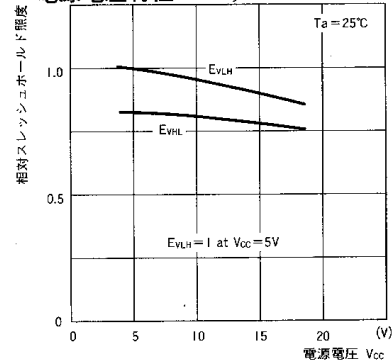
■相対スレッショールド照度/ 電源電圧特性 EVLH, EVHL/VCC
