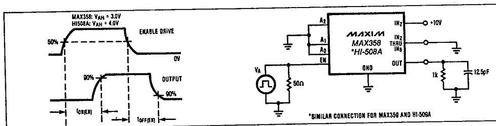
Figure 3. Enable Delay ( t_{ON(EN)} , t_{OFF(EN)} )
