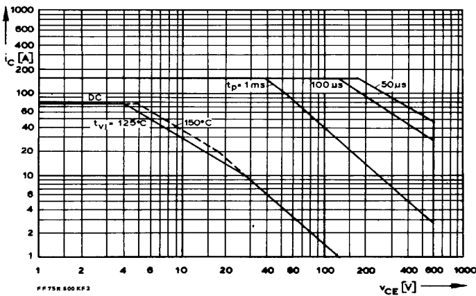
3 Vorwärts-Arbeitsbereich FBSOA (Einzelpuls, nicht periodisch). Forward biased safe operating area (single pulse, non repetitive). t_C = 25^\circ\text{C}
