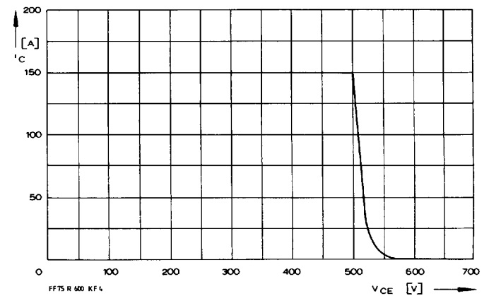
4 Rückwärts-Arbeitsbereich RBSOA. Reverse biased safe operating area. t_{vj} = 125^\circ\text{C} , V_{LF} = V_{LR} = 15\text{ V} , R_G = 33\ \Omega
