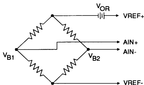
Figure 6. VOR Offset
