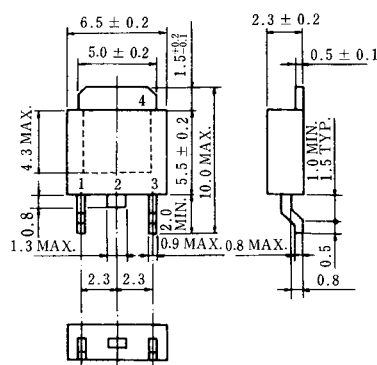
2SB1261-Z外形図
