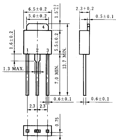
2SB1261外形図
