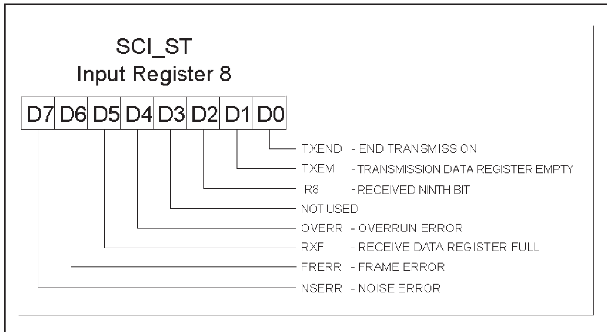
Figure 2.7. SCI_ST Registers
