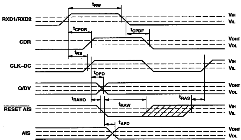
Fig. 7 Decoder timing parameters
