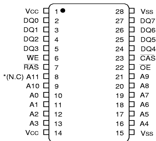
28Pin Plastic SOJ (300mil)
