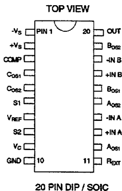
20 PIN DIP / SOIC
