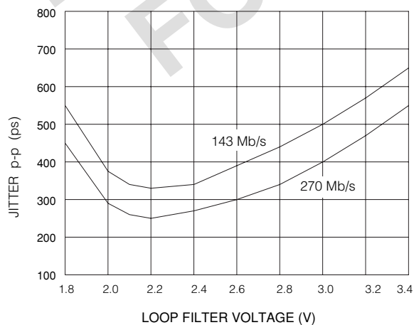
Fig. 16 Output Jitter
