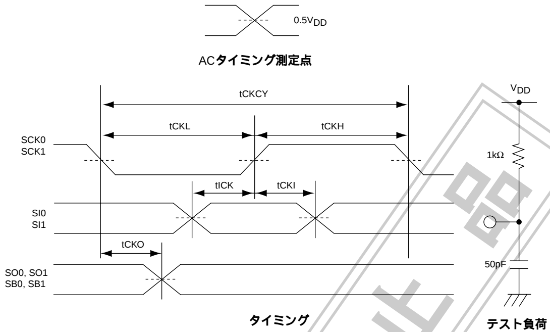
図6 シリアル入出力テスト条件
