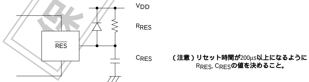
図5 リセット回路
